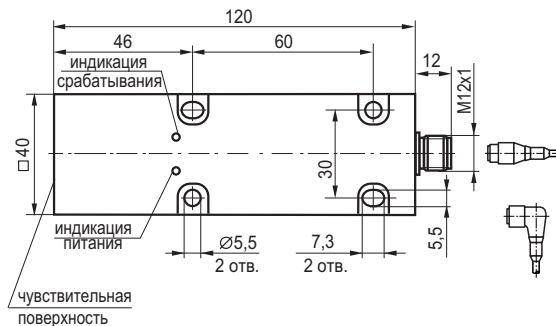
Габаритный чертёж
